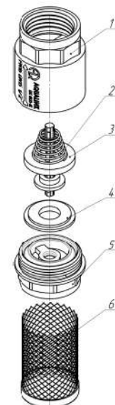
Рисунок 2 – Общий вид и конструкция изделия
