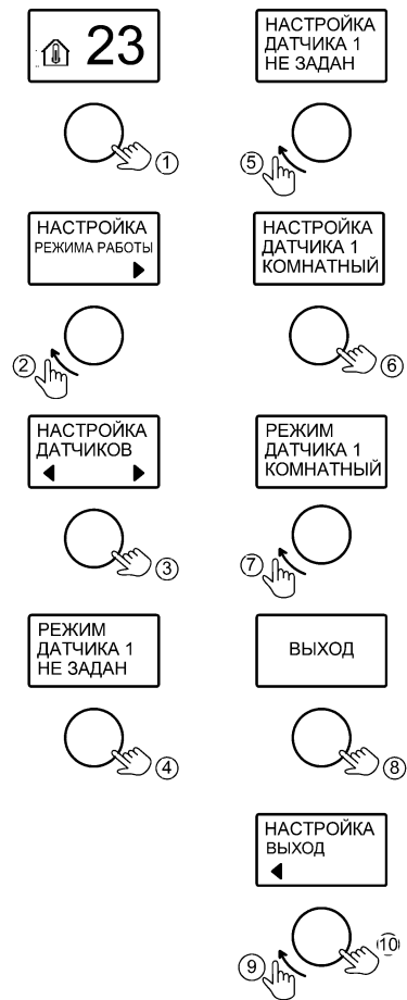
Рисунок 11. Настройка датчиков температуры воздуха
